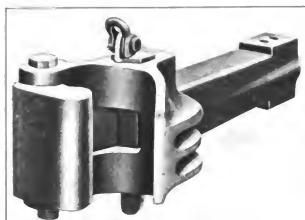
Fig. 3967. R. E. Janney Coupler.
